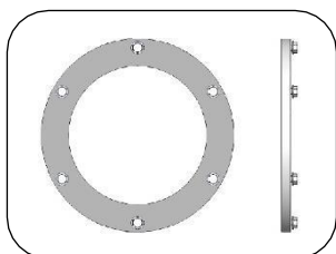
SUPORTE FLANGE PARA CILINDROS LS-15 / LS-20
