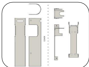
SUPOORTE PARA ATUADOR PNEUMÁTICO - 2º DISPARO
