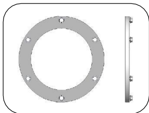
SUPORTE FLANGE PARA CILINDROS, LS-10 / DCS-68 (10 GAL)
